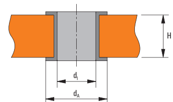
PCB parameters
